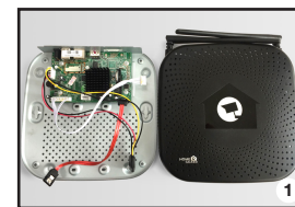
Odpojte NVR od napájení, vyšroubujte šroubky a sejměte horní kryt.
