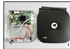
Odpojte NVR od napájania, vyskrutkujte skrutky a zložte horný kryt.
