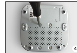
Pomocí šroubků uchyťte disk HDD ze spodní strany rekordéru. Nasuňte horní kryt a upevněte šroubky.
